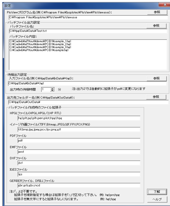
PloViewAuto 設定画面
